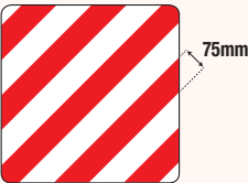
Overlastbord: 500x500mm - PP en Alu voorzien van 2 boringen - Folie klasse I Panneau charges exédentaires: 500x500mm - PP et Alu prévus de 2 trous - Film classe I
