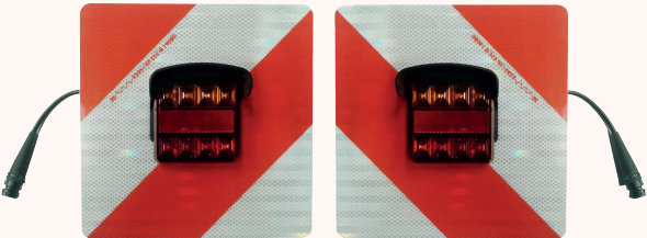
Overlastborden met LED systeem - Enkelzijdig folie Met weerstand gemonteerd - LED 12V + 7 mtr. kabelset Voor bevestiging op de achterzijde
