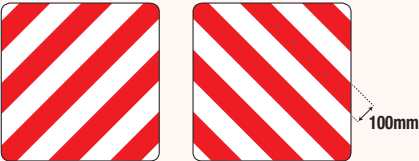
Overlastbord: 423x423mm - Zonder boringen - Folie klasse II Panneau charges exédentaires: 423x423mm - Sans trous - Film classe II
