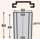
Steun in gegalvaniseerd staal Support en acier galvanisé
