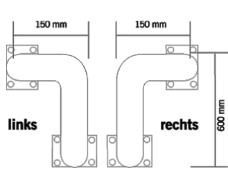
Hoekbeugel enkelzijdig, verdiepte uitvoering voor vloermontage
